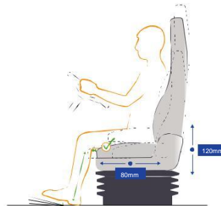
Réglage pneumatique avancé de la hauteur (120 mm) et de la profondeur d'assise (80 mm) Advanced pneumatic height adjustment (120 mm) and seat cushion depth adjustment (80 mm)
